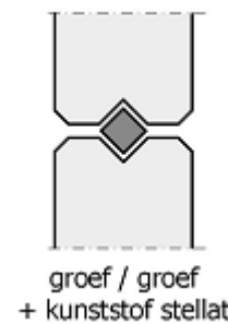
Details onderlinge aansluiting
